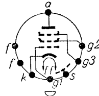
Sockelschaltenschema
